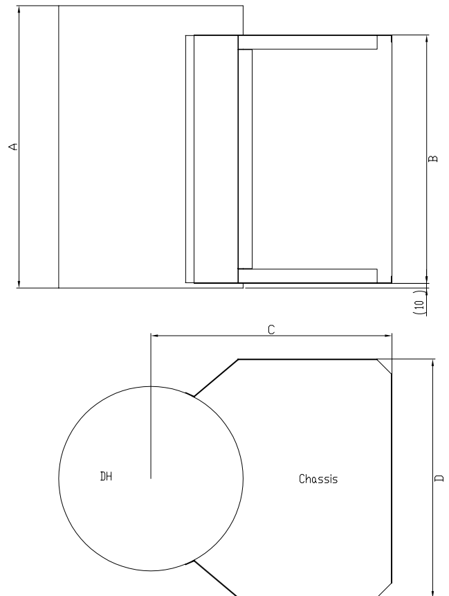
Maßskizze DDL15/15-25
